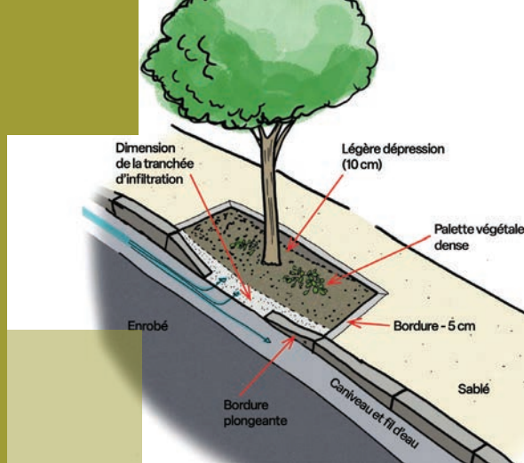
Schéma de principe d'un « arbre de pluie »
