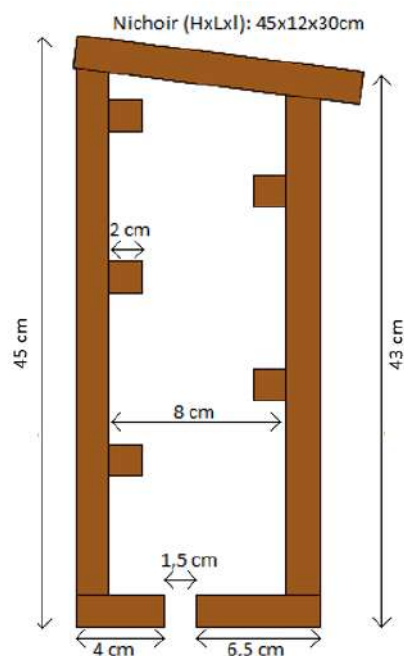
Plan d'un nichoir
